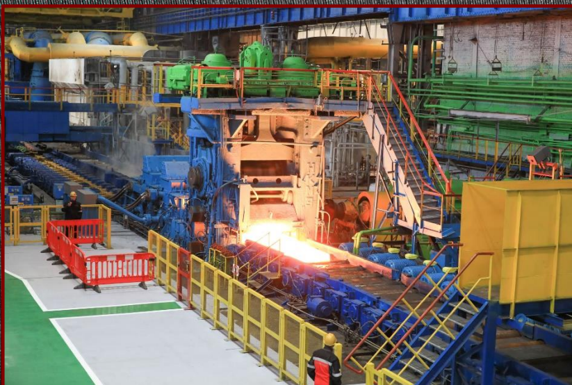
Листо-прокатный цех 1700 ЧАО “ММКИ”
