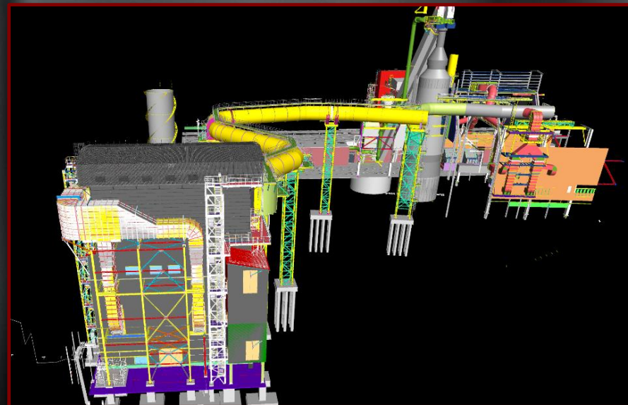
Газоочистка доменной печи №4 ЧАО "ММКИ"
