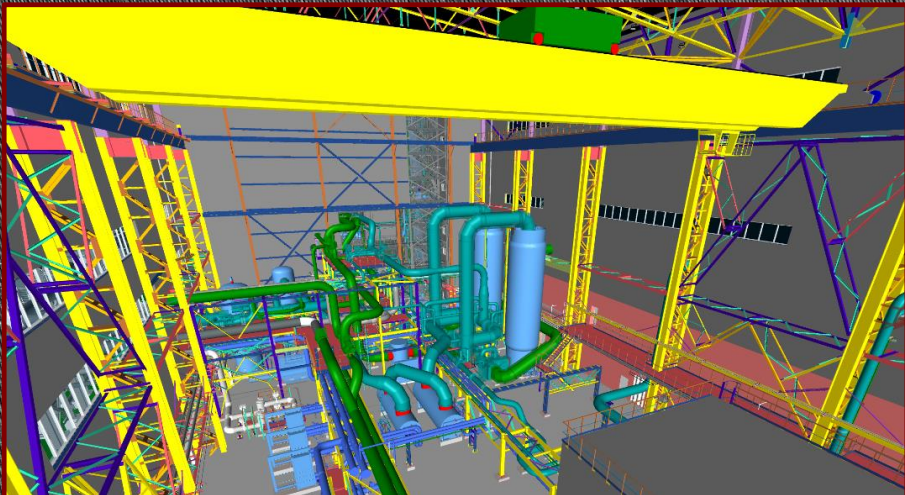
Установка разделения воздуха на ЧАО "ММКИ"
