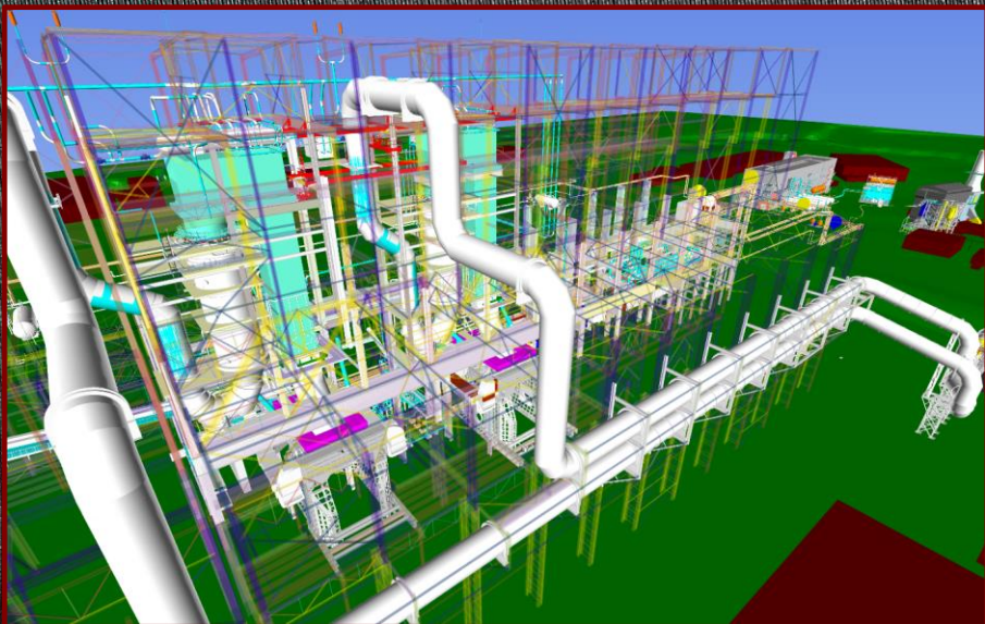
Реконструкция системы газоочистки ККЦ ЧАО "МК "АЗОВСТАЛЬ"
