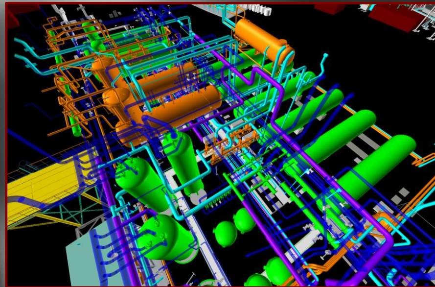
Модернизация энергоблока ККЦ ЧАО "МК "АЗОВСТАЛЬ"
