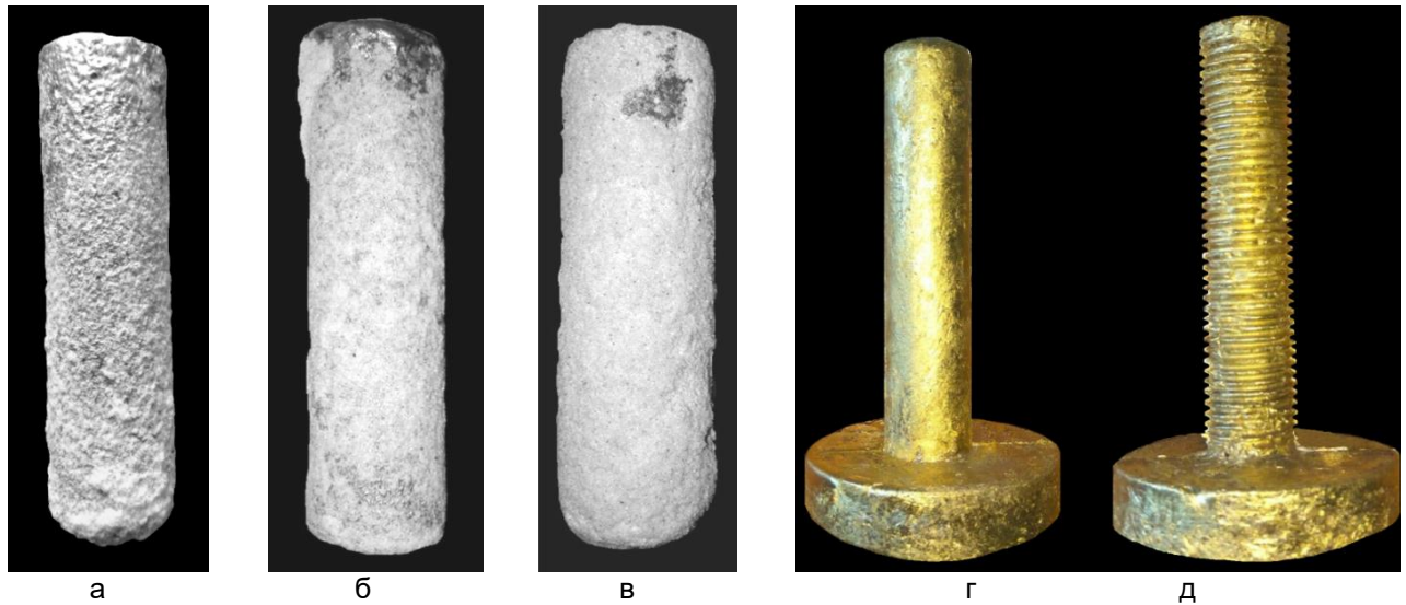
Рисунок 6. Вигляд зразків з бронзи БрО3А3 (а), БрО5Ц5С5 (б), БрА9Ж3Л (в) після вибивання з ПРФ форми та зразків з бронзи БрА3О3, відлитих в гладкий (г) та ребристий (д) кокіль
