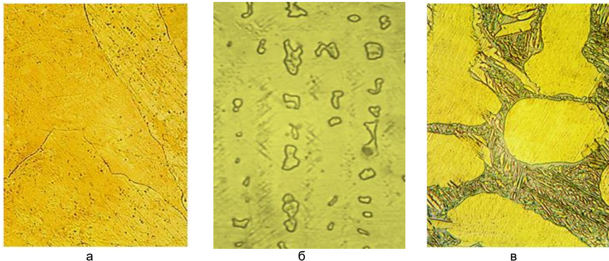
Рисунок 5. Мікроструктури ( \times 1000 ) бронз з величиною K_x=2,4 (а), K_x=4,9 (б), K_x=7,6 (в)
