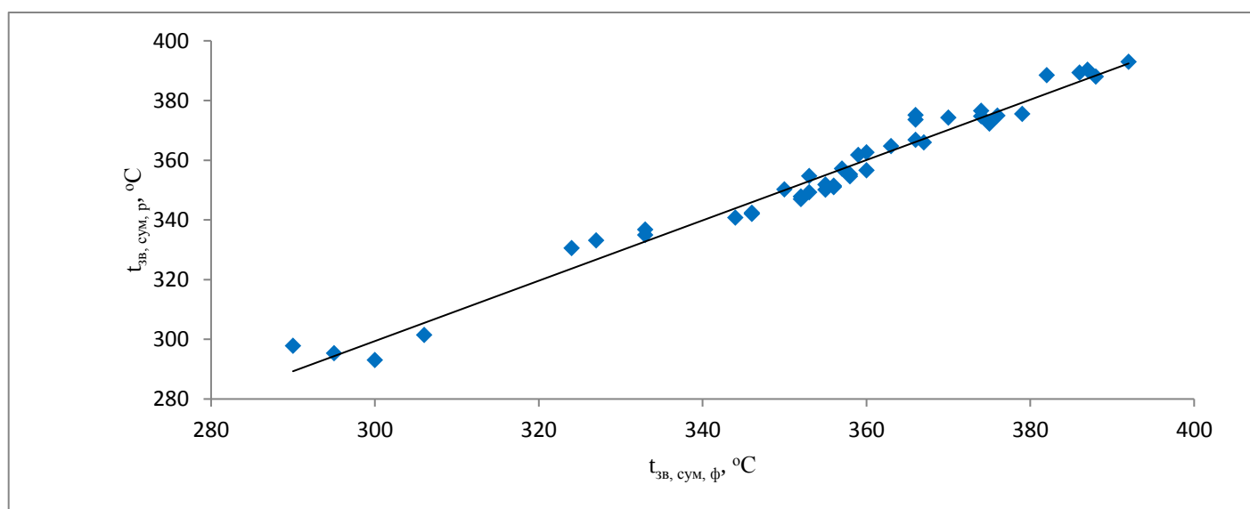
Рисунок 3.2 – Залежність між фактичними і розрахунковими значеннями температур займання бінарних сумішей (в співвідношенні 50:50).
