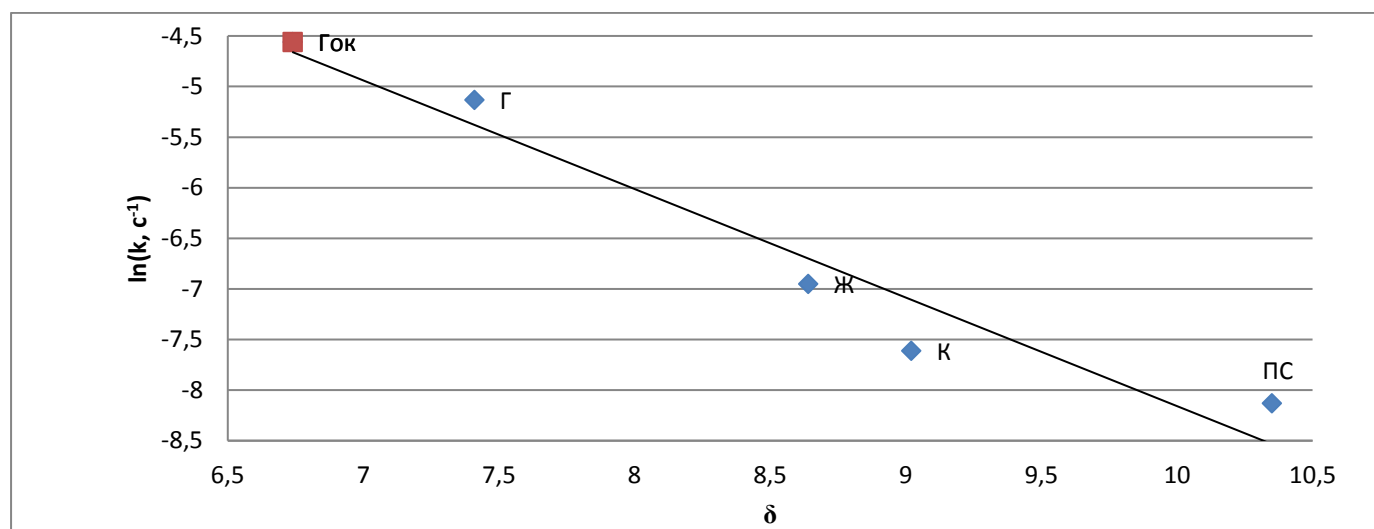
Рис. 4.4 – Залежність константи швидкості займання при 350°C від структурного параметра \delta
