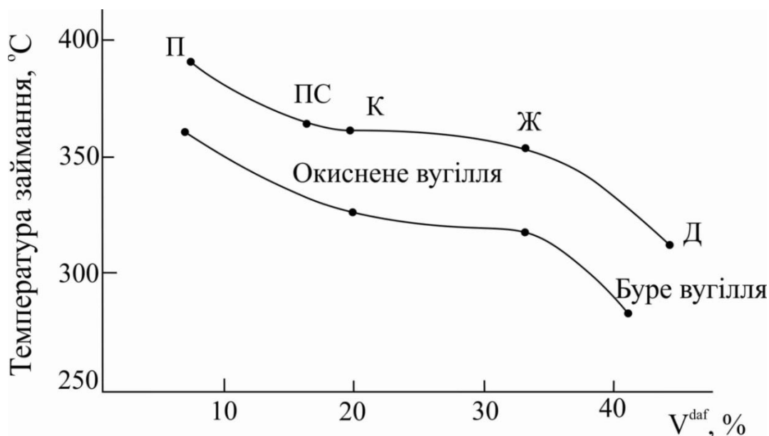
Рисунок 2.2 – Зниження температури займання при окисненні вугілля різного ступеня метаморфізму
