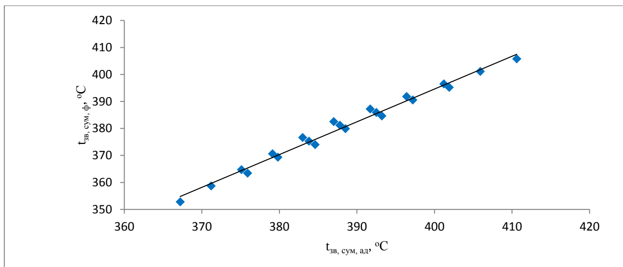
Рисунок 3.8 – Залежність між значеннями температур займання модельних трикомпонентних сумішей, розрахованих за правилом адитивності і за рівнянням (3.5)
