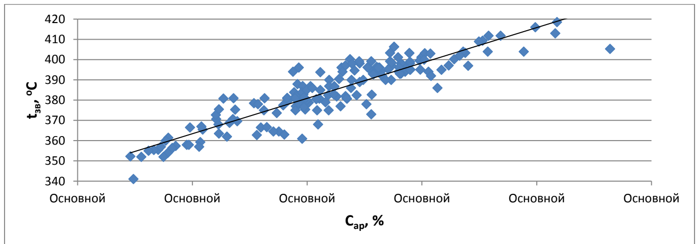
Рисунок 5.5 – Залежність t_{3в} від C_{ар}
