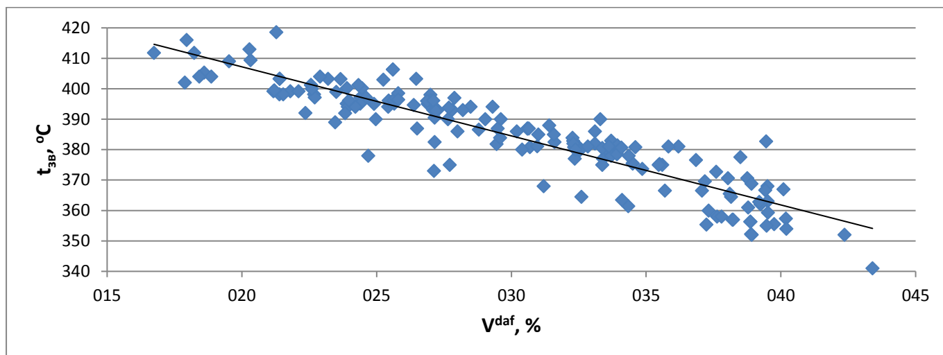
Рисунок 5.1 – Залежність t_{3B} від V^{daf}
