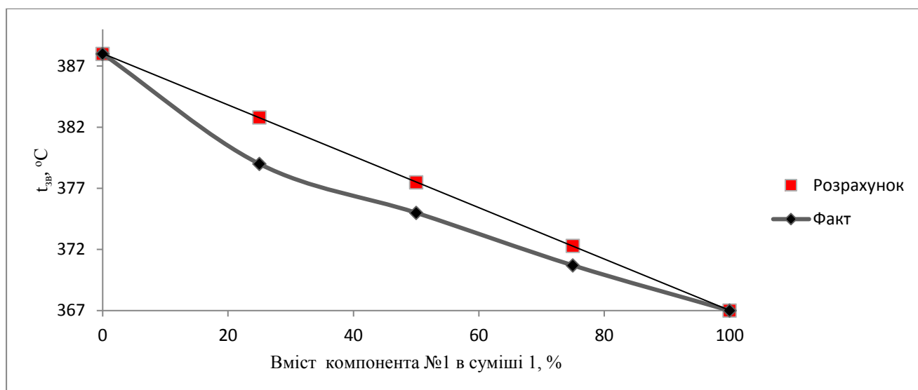
Рисунок 3.3 – Фактичні і розрахункові значення t_{зв} суміші 1
