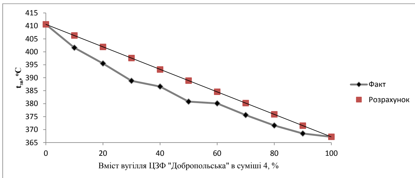
Рисунок 3.6 – Фактичні і розрахункові значення t_{зв} суміші 4.
