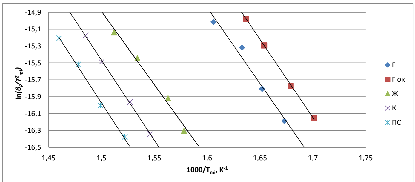
Рисунок 4.2 – Залежність \ln(\beta_i/T_{mi}^2) від 1000/T
