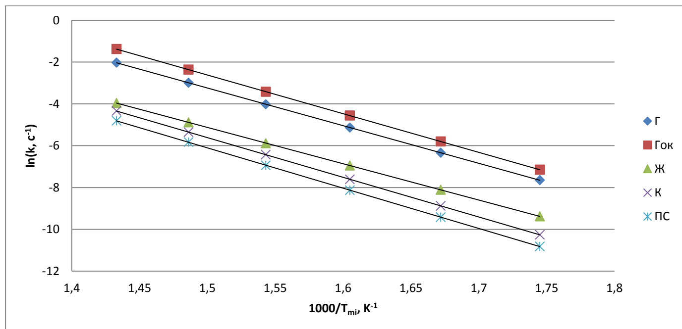
Рисунок 4.3 – Залежність константи швидкості від температури займання
