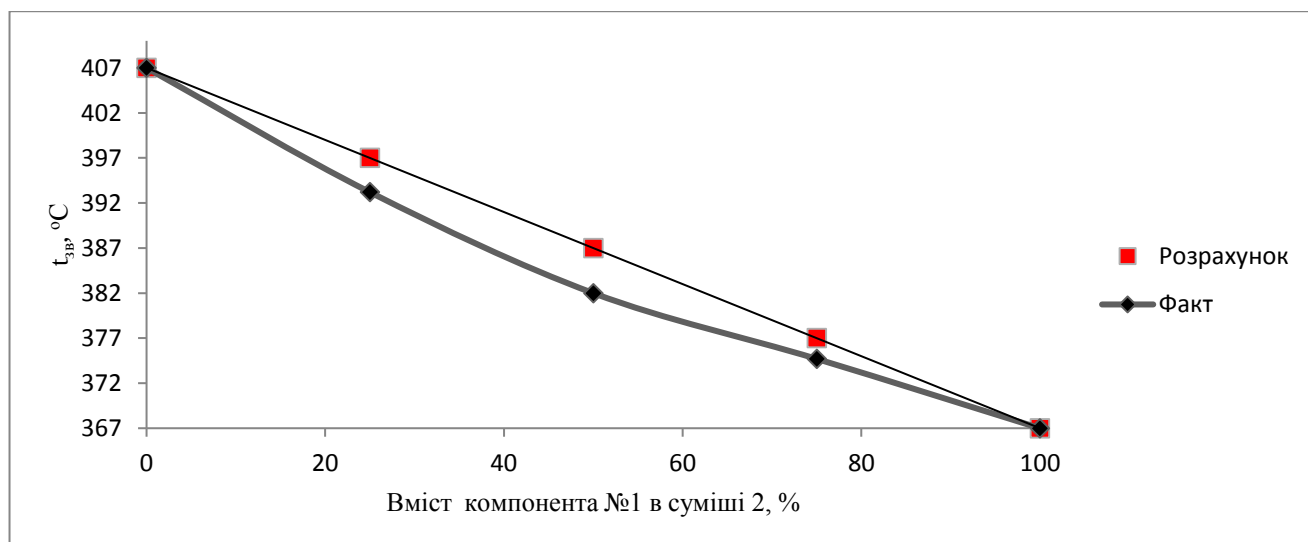
Рисунок 3.4 – Фактичні і розрахункові значення t_{зв} суміші 2
