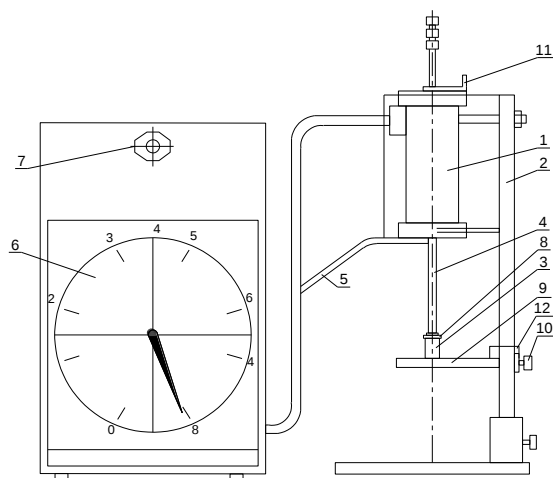
Рисунок 1.2 – Устаткування для модифікованого комплексного методу прикоксовування
