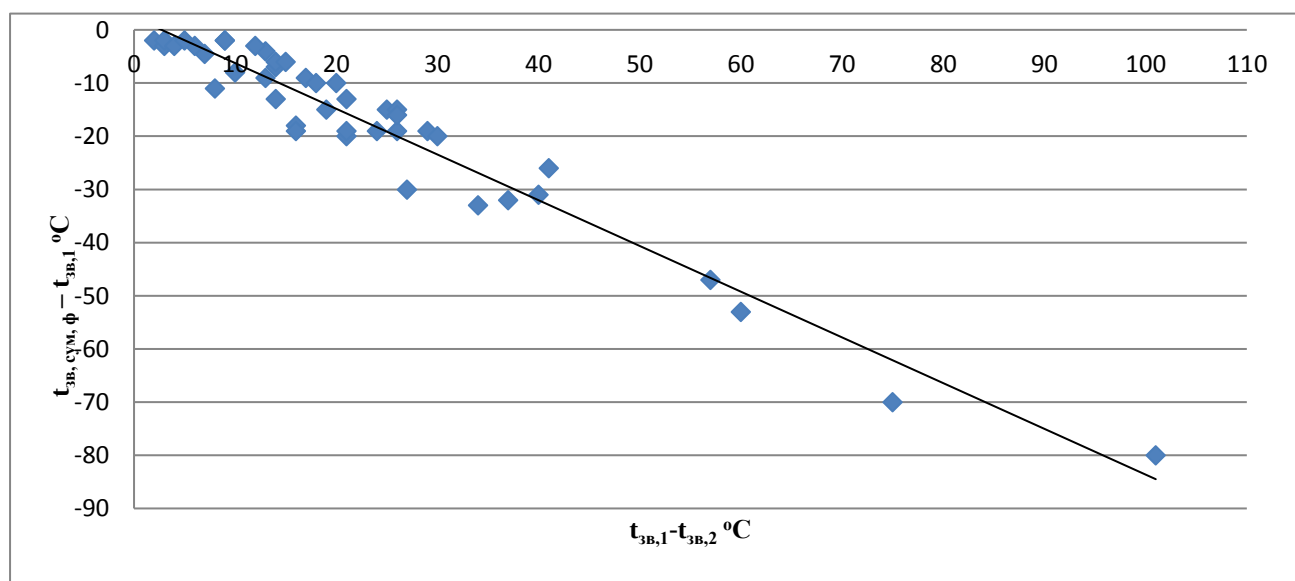
Рисунок 3.1 – Залежність t_{зв, сум, ф} - t_{зв,1} від t_{зв,1} - t_{зв,2}
