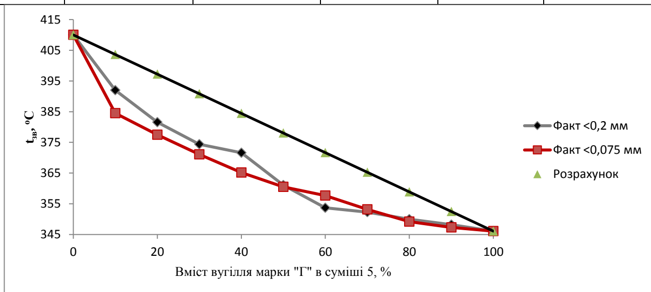
Рисунок 3.7 – Фактичні і розраховані значення t_{зв} суміші 5
