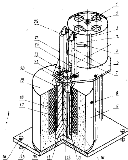
Рисунок 1.1 – Дилатометр ІГК-ДМетІ
