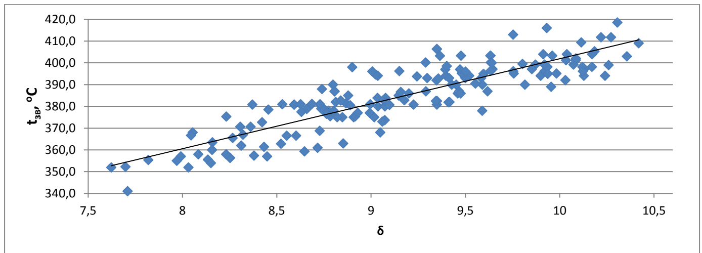
Рисунок 5.4 – Залежність t_{3в} від \delta
