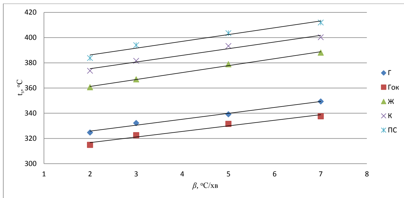
Рисунок 4.1 – Графічна залежність температури займання від швидкості нагріву вугілля різних марок і ступеня окиснення
