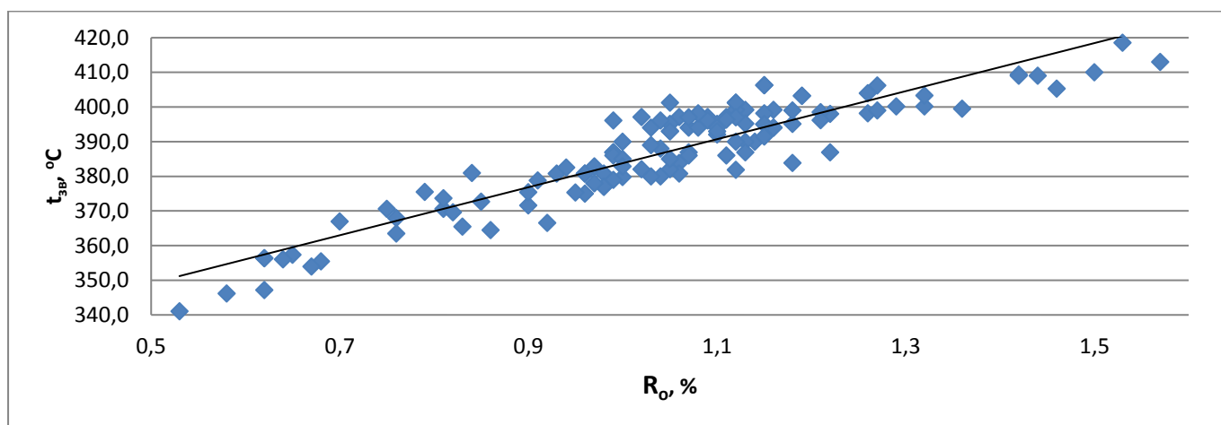
Рисунок 5.2 – Залежність t_{3B} від R_0
