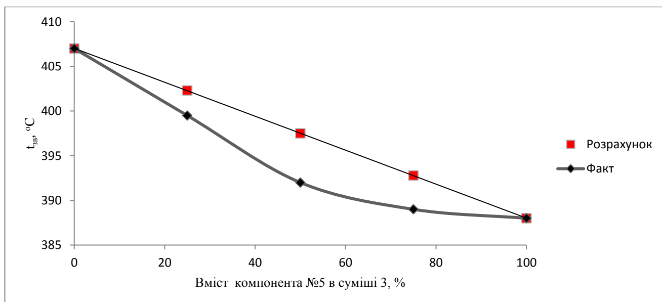
Рисунок 3.5 – Фактичні і розрахункові значення t_{зв} суміші 3
