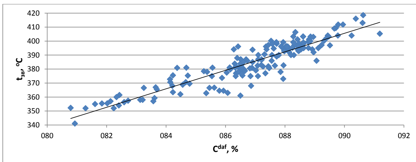
Рисунок 5.3 – Залежність t_{3B} від C^{daf}
