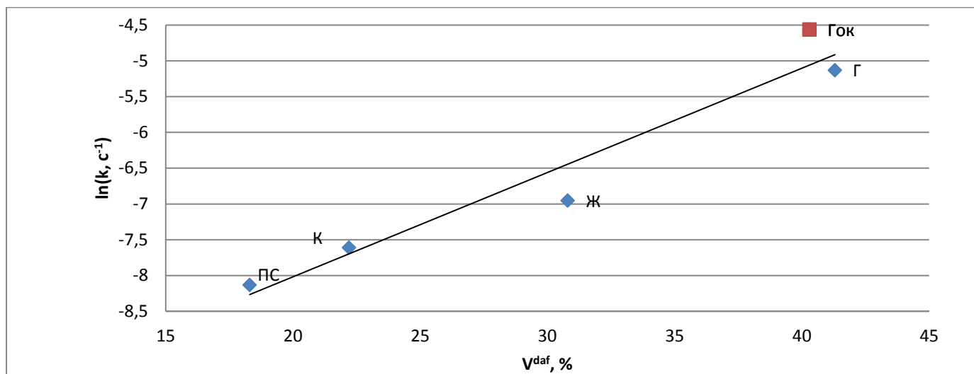
Рисунок 4.5 – Залежність константи швидкості займання при 350 °C від виходу летких речовин
