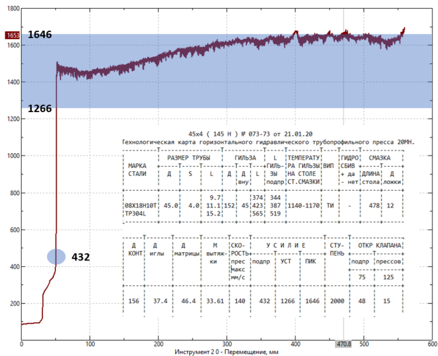
Мал. 10 – Графік розподілу сили пресування залежно від переміщення голки для труби 45x4 мм
