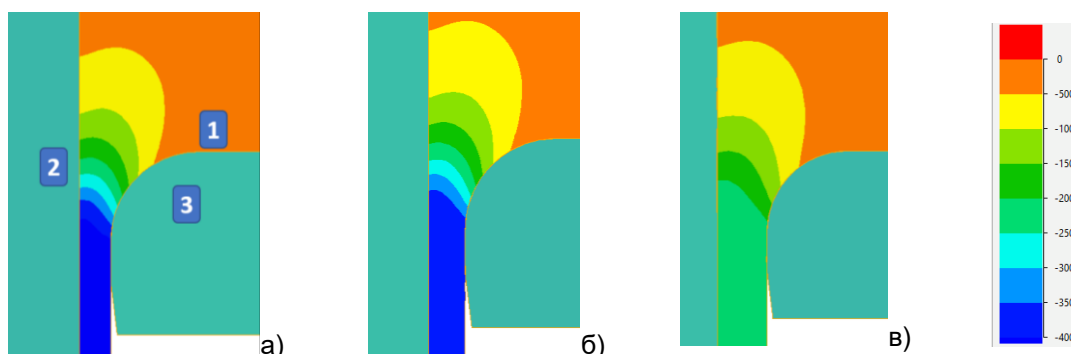
Рис.18.-Розподіл швидкості закінчення металу в осередку деформації для труб розмірами: а - 45х4 мм; б - 45х4, 5 мм; в - 88,9 х6, 45 мм (де: 1 - гільза, 2 - голка, 3 - матриця).
