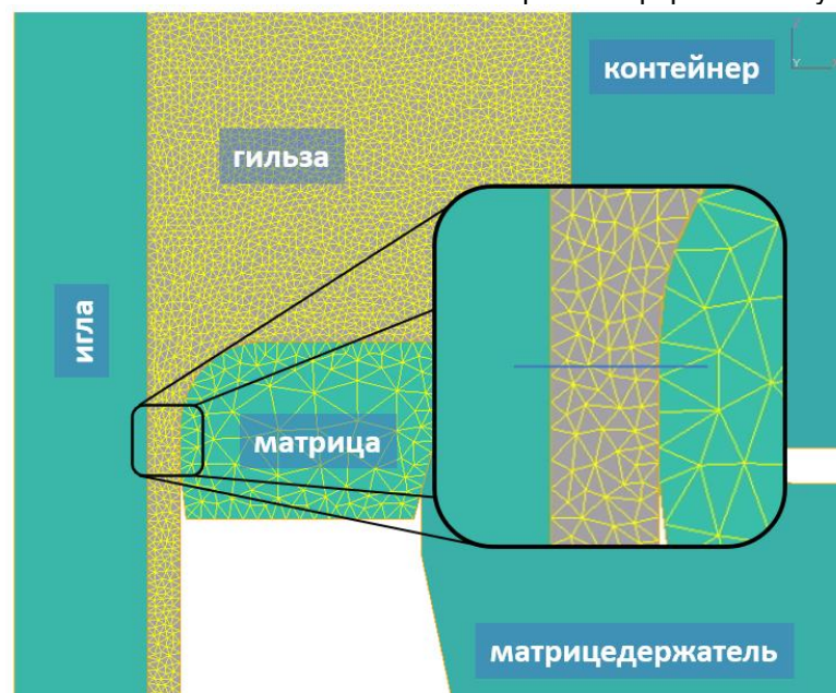
Мал. 8 – Розбивка гільзи на кінцеві елементи
