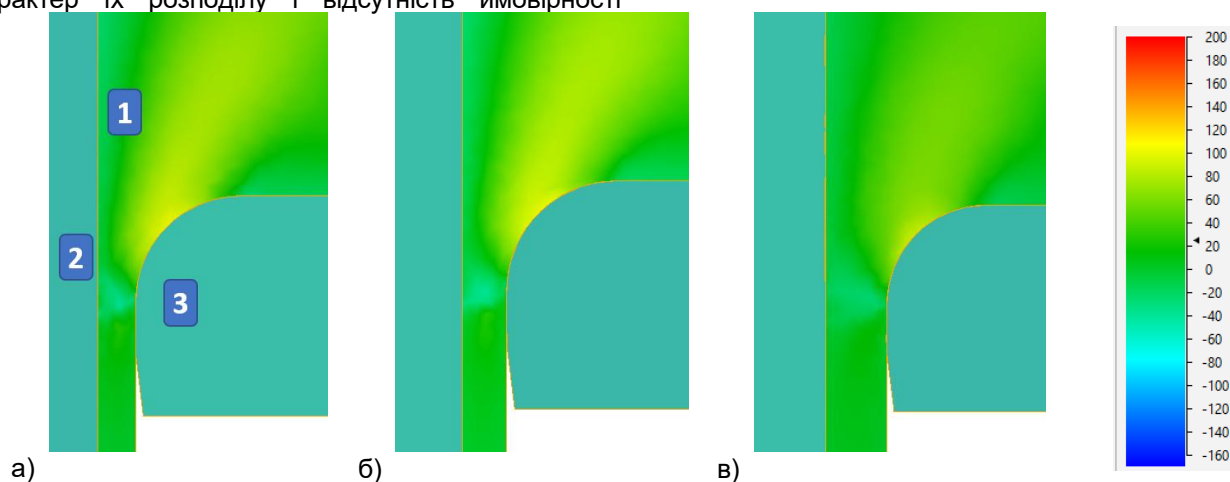
Мал. 22 – Розподіл дотичних напруг в осередку деформації для труб розмірами: а – 45x4 мм; б – 45x4, 5 мм; в – 88,9x6,45 мм (де: 1 – гільза, 2 – голка, 3 – матриця)
