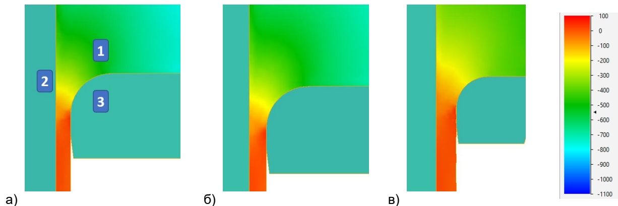
Рис. 14 . розподіл середньої напруги в осередку деформації для труб розмірами: а – 45x4 мм; б - 45x4, 5 мм; в - 88,9 х6, 45 мм (де: 1 - гільза, 2 - голка, 3 - матриця).
