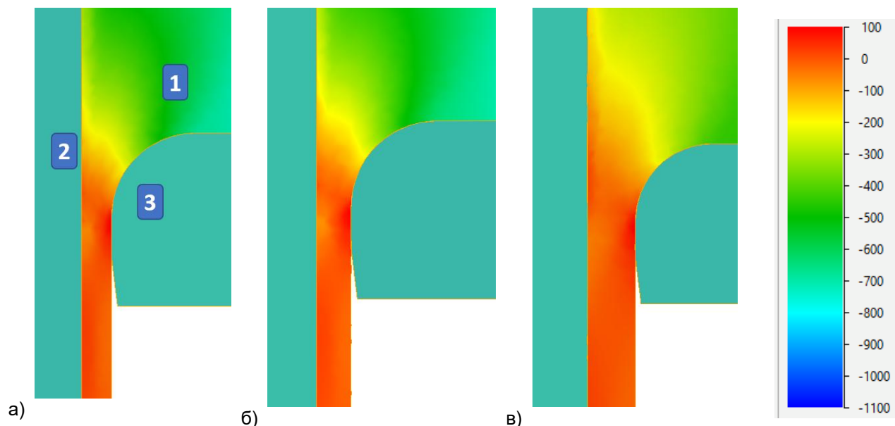
Мал. 20 – Розподіл нормальних напруг в осередку деформації для труб розмірами: а – 45x4 мм; б - 45x4, 5 мм; в – 88,9x6,45 мм (де: 1 – гільза, 2 – голка, 3 – матриця)
