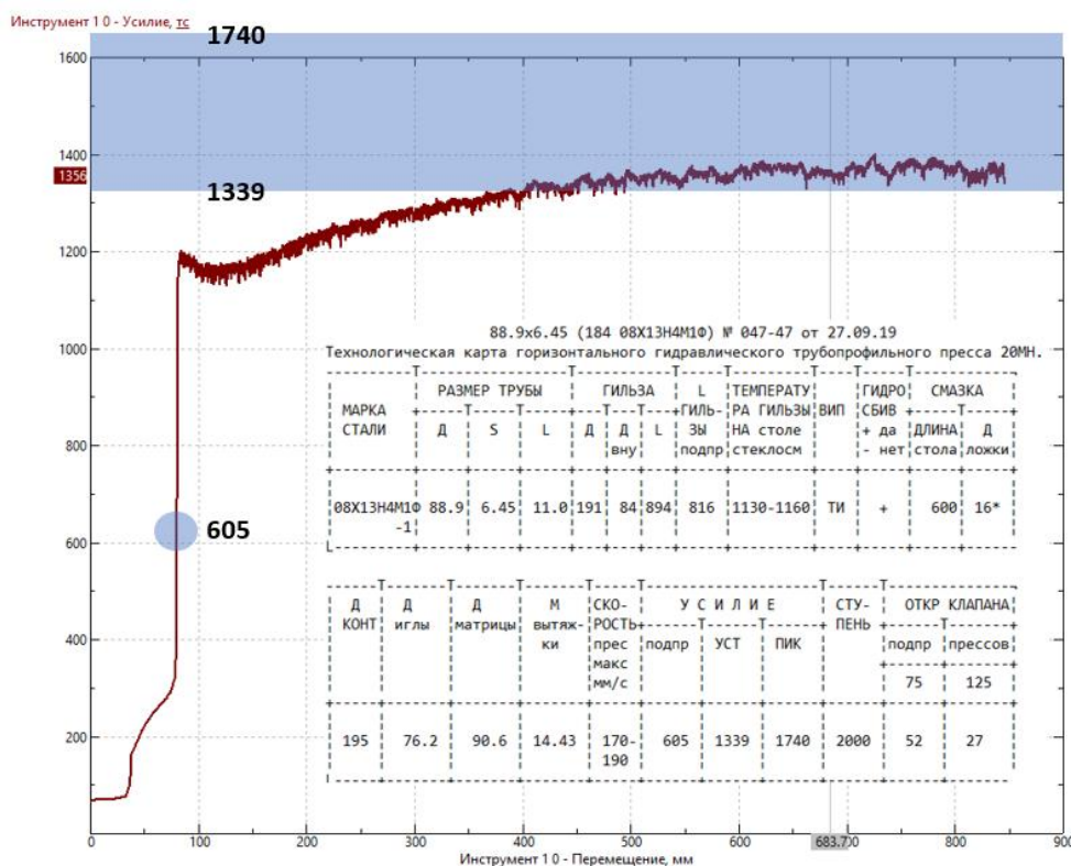
Мал. 12 – Графік розподілу сили пресування, залежно від переміщення голки для труби. 88,9 х 6, 45 мм
