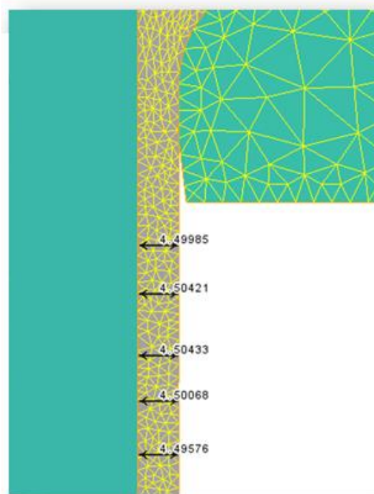
Мал. 9 – Товщина стінки труби 45x4 мм у ПП QForm .
