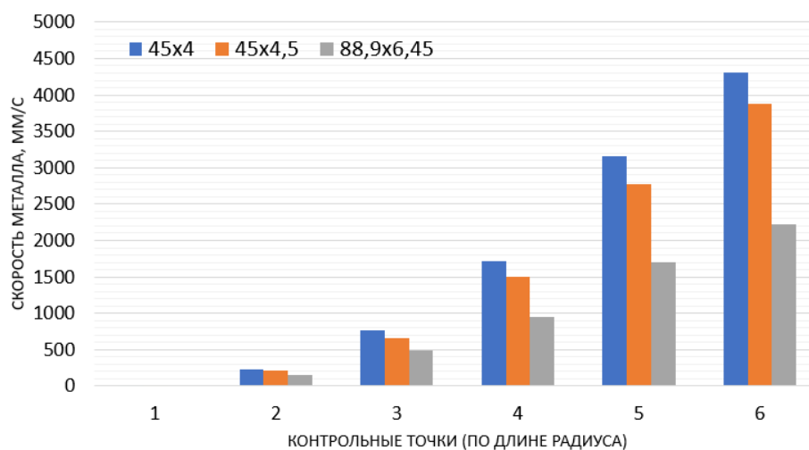
Малюнок 19 – Графік розподілу швидкості витікання металу.
