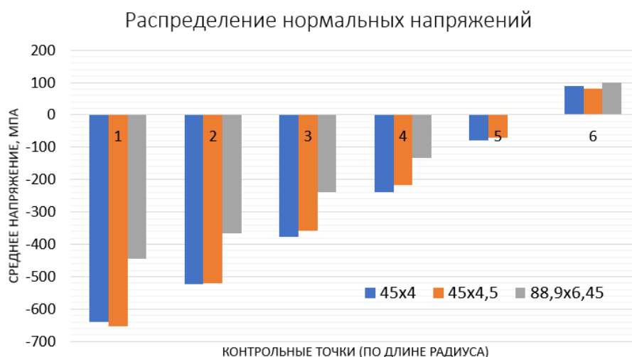
Малюнок 21 - Графік розподілу нормальних напруг
