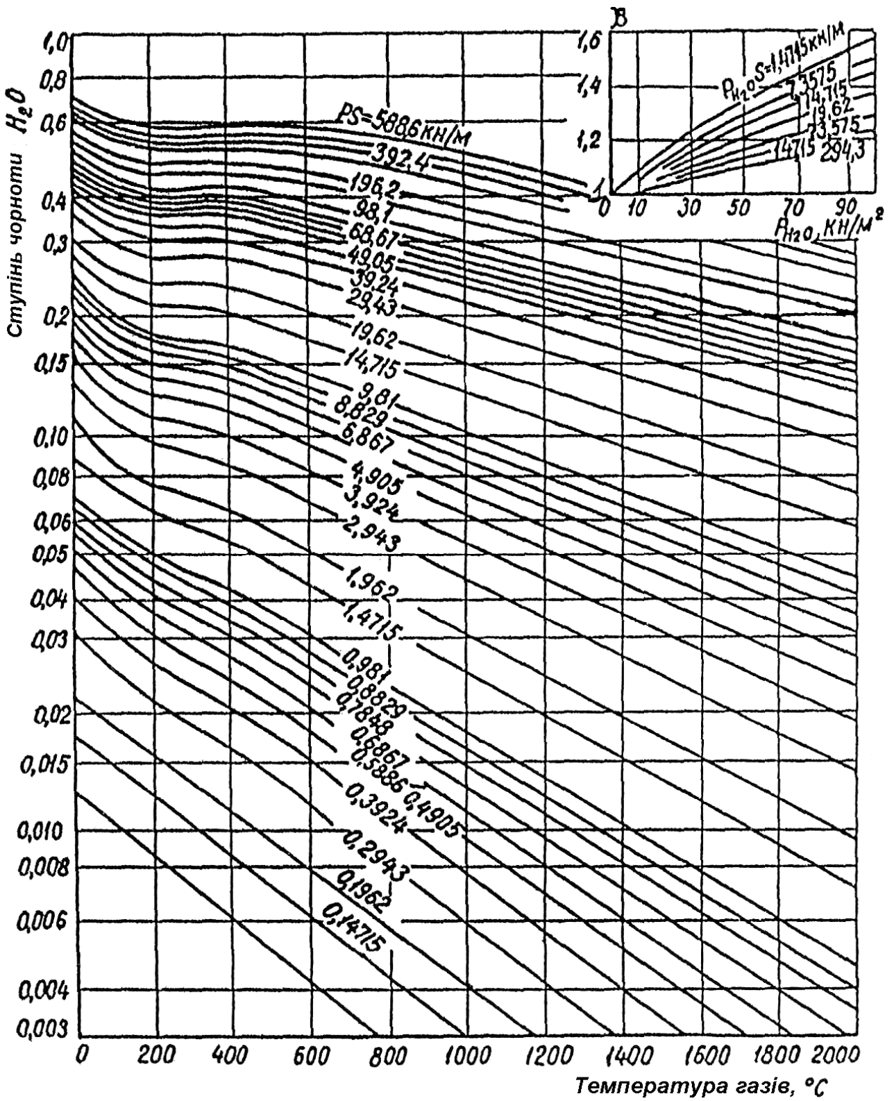
Рисунок 2.4 б – Ступінь чорноти при випромінюванні H 2 O
